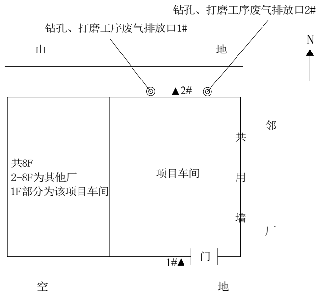
图 3-2 厂区平面布置及监测点位
