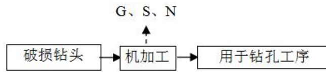
图 3-4 项目钻头生产工艺及产污环节流程图
