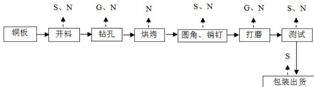
图 3-3 项目铜板生产工艺及产污环节流程图
